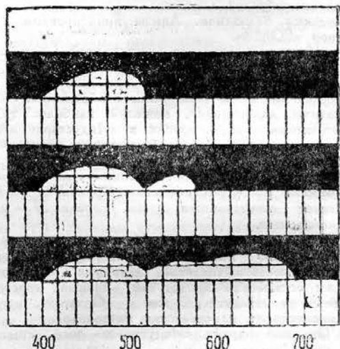
Рис. 2. Спектральная чувствительность А—простых пластинок, В—ортохроматических пластинок, С—панхроматических пластинок
