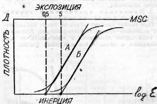
Рис. 6. Определение кратности светофильтра по ХД. На рисунке: А — кривая, полученная без светофильтра, Б — кривая со светофильтром
