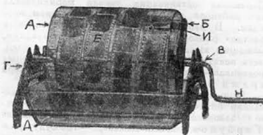
Рис. 19. Проявительный цилиндр
